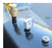
Indicatore di livello visivo e filtro ai carboni attivi. Mechanical level gauge and activated carbons vent filter.
