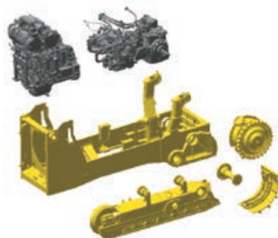
Treno di potenza modulare
