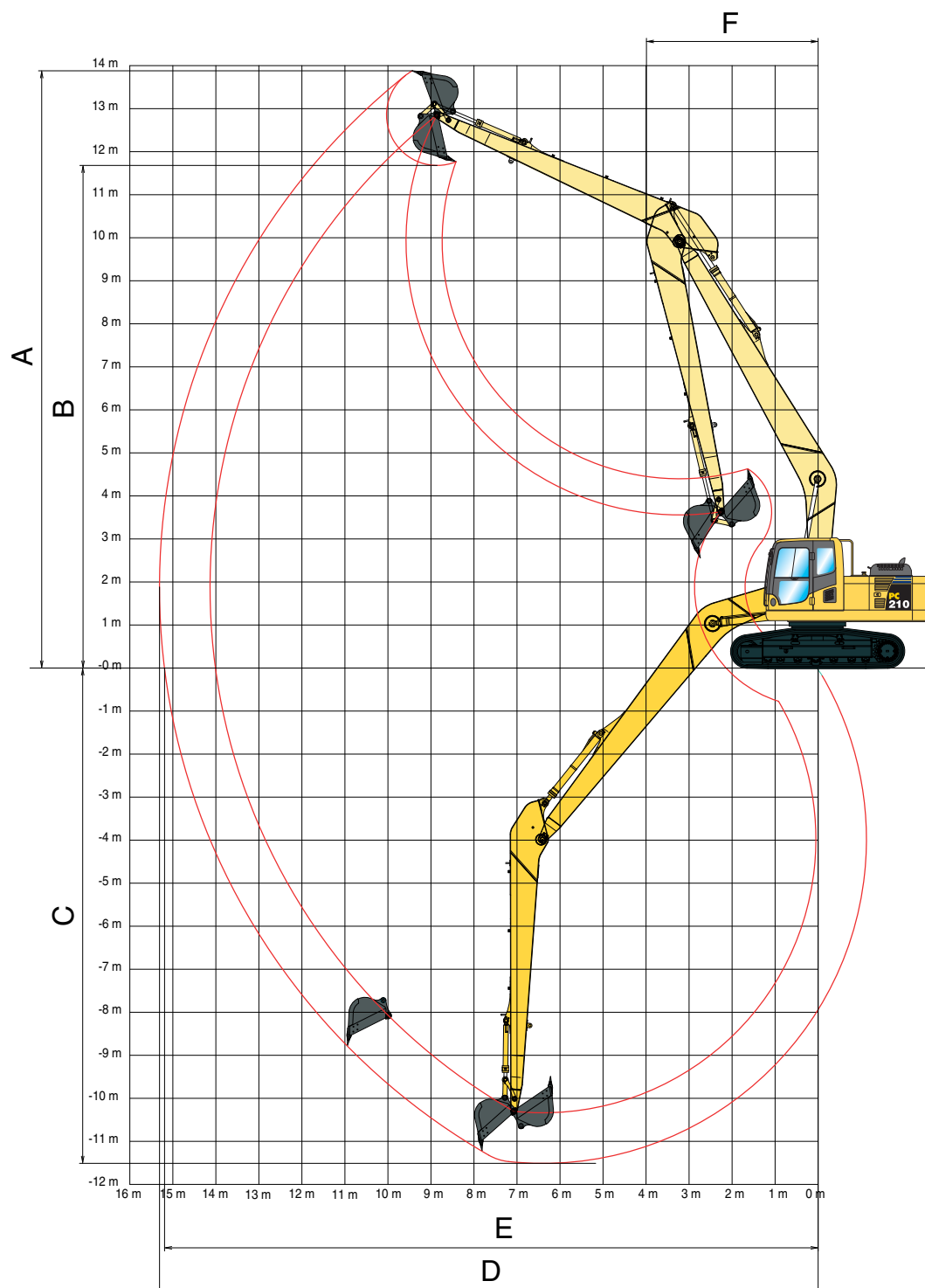
Diagramma di scavo PC210LC/NLC-8 Super Long Front
